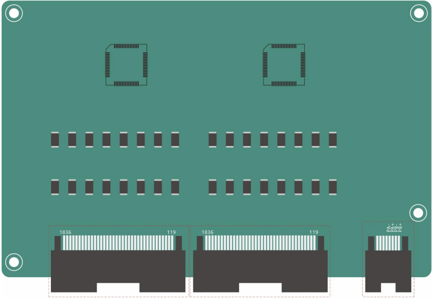
J1:采样端口-1
