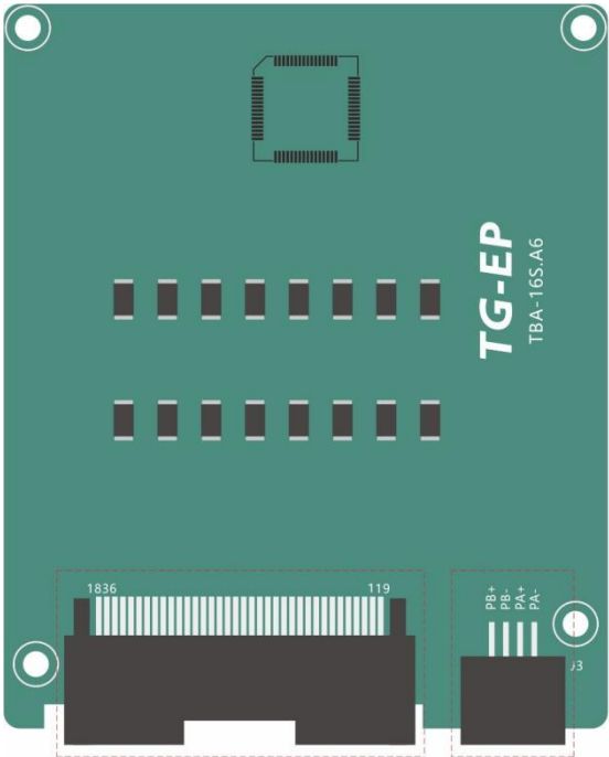
J1:采样端口 J3:菊花链通讯
